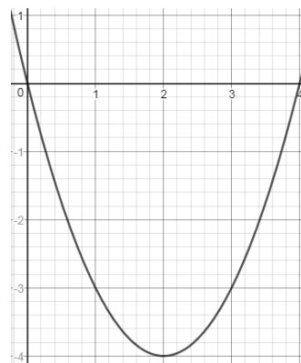
г) D(y): (-\infty; -1] \cup (-1; \infty) , общий вид
