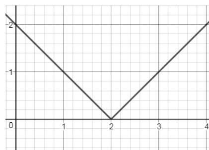
в) D(y): \mathbb{R} , общий вид
