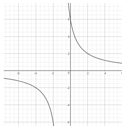
д) D(y): \mathbb{R} , общий вид
